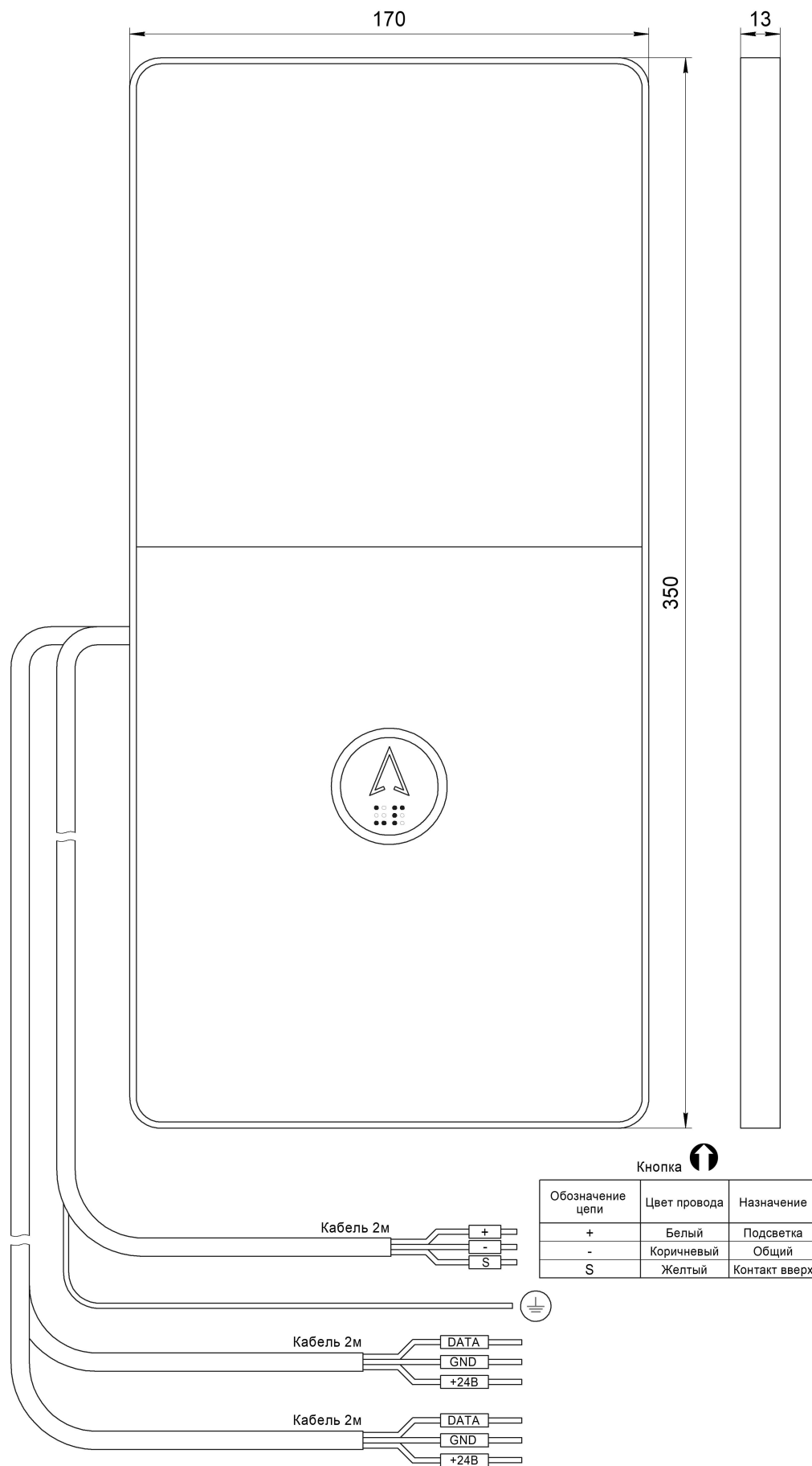
Рис.1 Внешний вид, габаритные и установочные размеры Вызывного поста МАЛАХИТ НШЕК.468381.076
